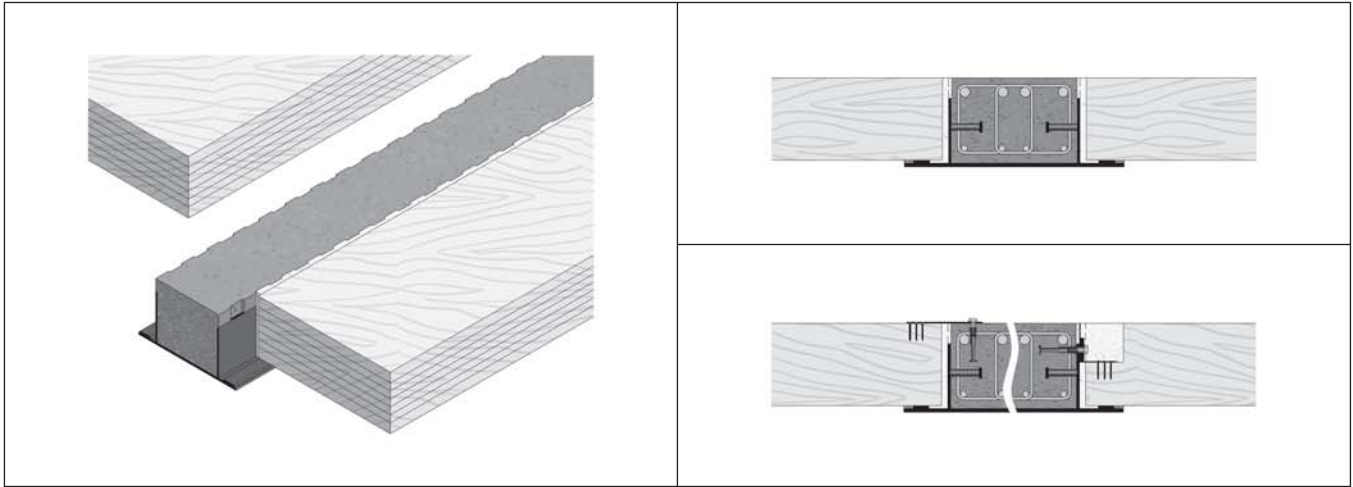
Holzbalkendecken. Holztafeln.
