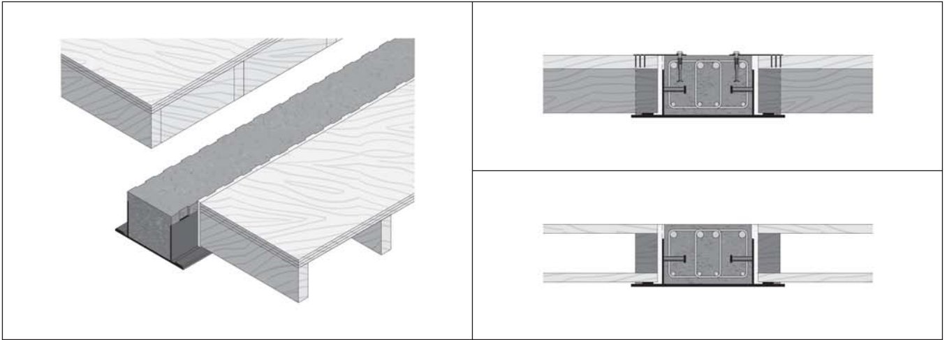
Holzbalkendecken. Holzrippen.
