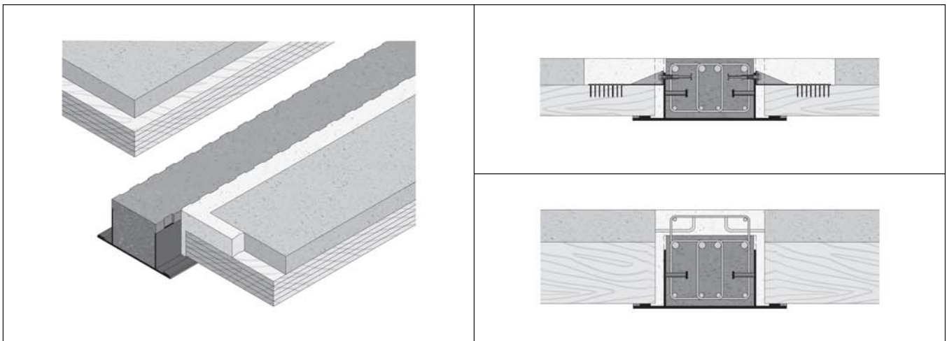
Holz-Beton-Verbunddecken (Betonfertigteilprofil), Holzplatten.
