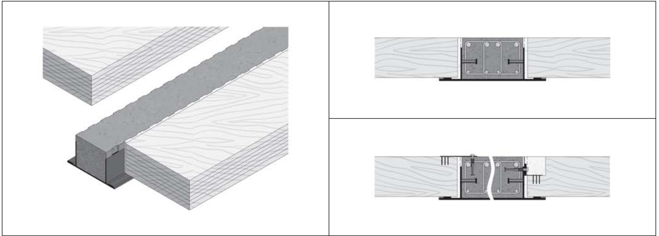
Holzbalkendecken. Holztafeln.
