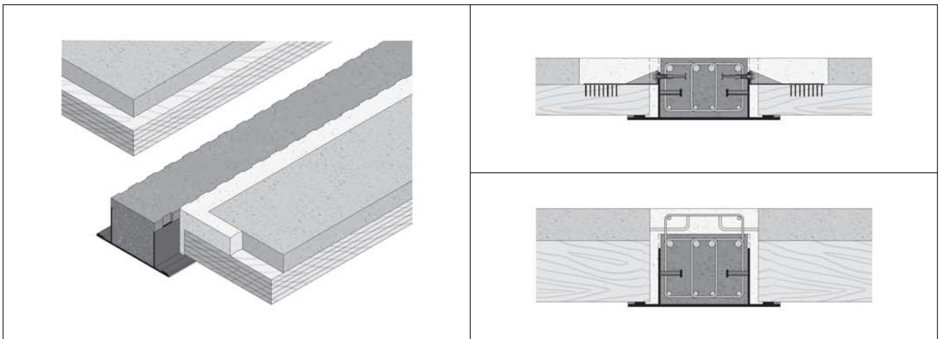
Holz-Beton-Verbunddecken (Betonfertigteilprofil), Holzplatten.
