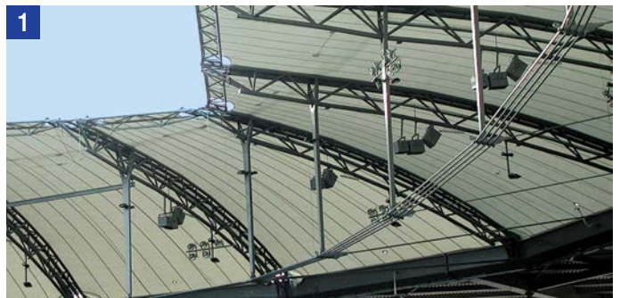
1 Ringseil mit unteren Speichenseilen und oberen Dreigurtbindern
