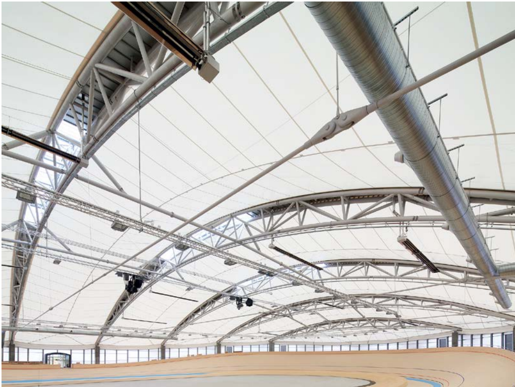
1 Zugstabsysteme mit Abhängung
