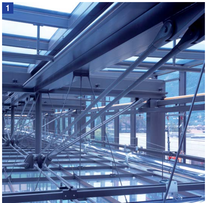
1 Unterspannung der Überkopfverglasung
